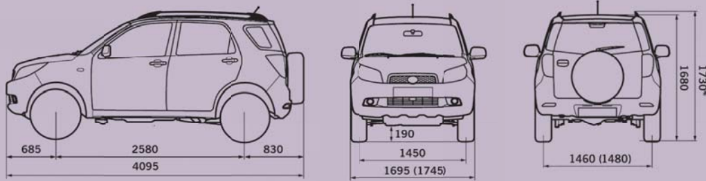
Alle Maße in mm. Angaben in Klammern zeigen Maße des Terios Top S. *Angabe für Terios 4WD.
